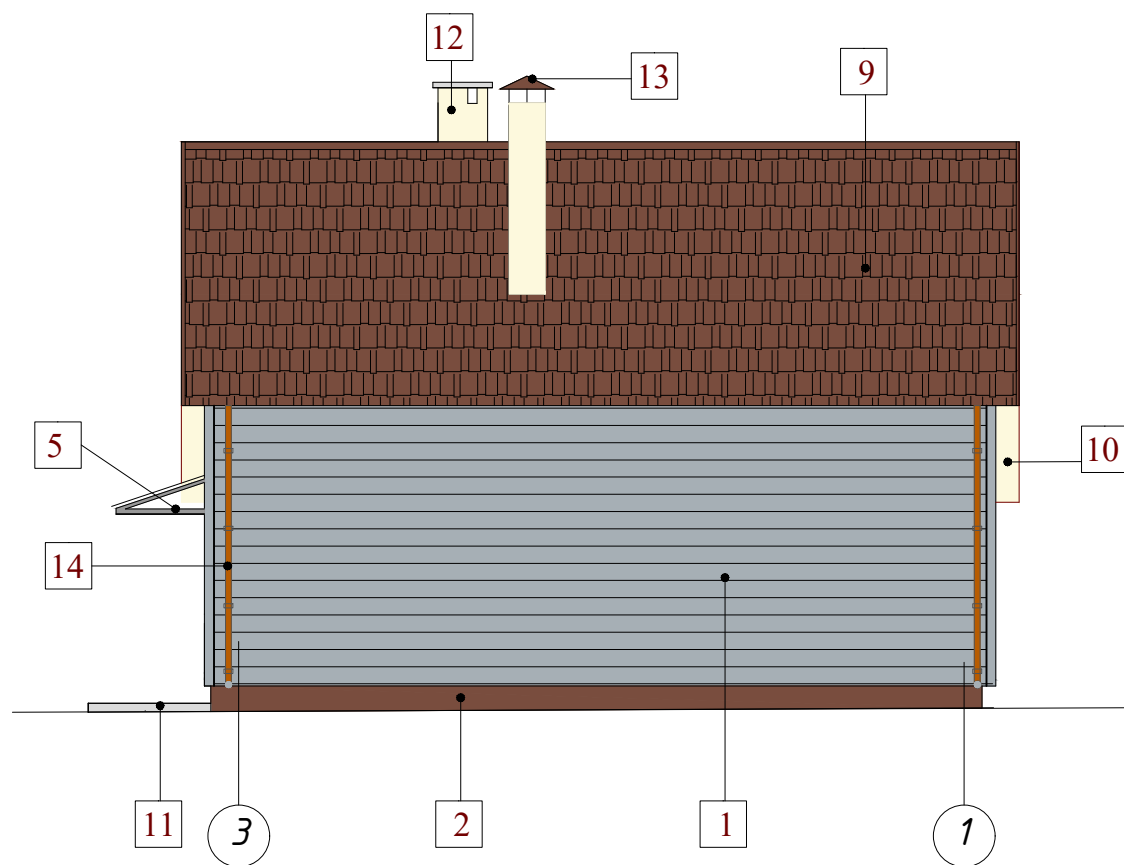
Фасад 3 - 1
