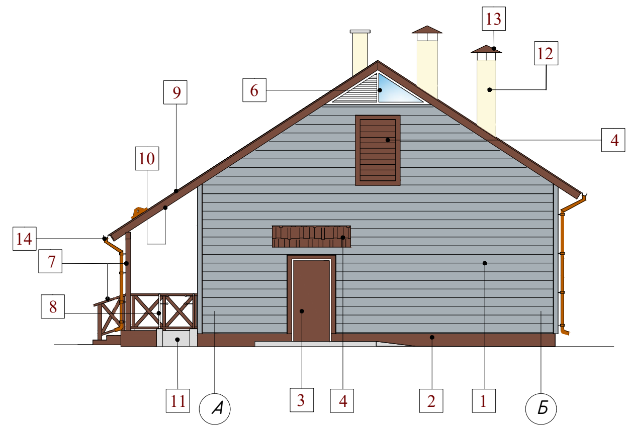
Фасад А - Б
