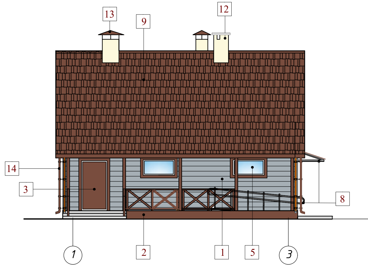
Фасад 1 - 3
